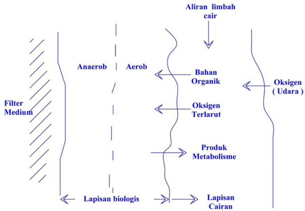
Gambar 16. Diagram proses biologis dalam filtrasi biologis
